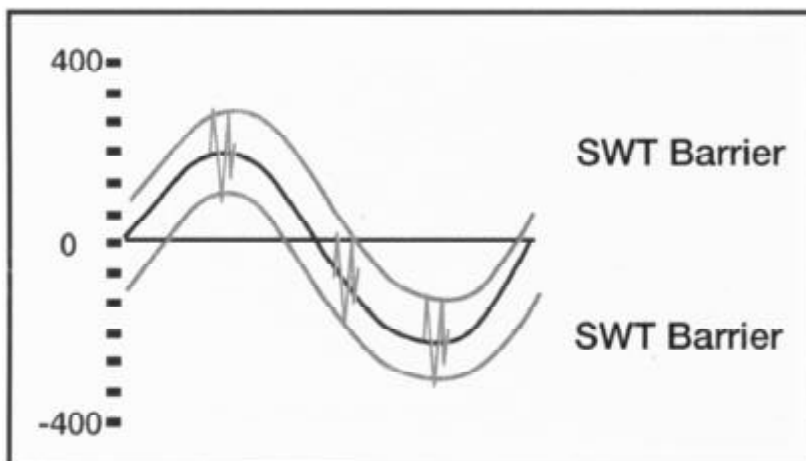
EFI:n transienttisuojat seuraavat siniaaltoa
